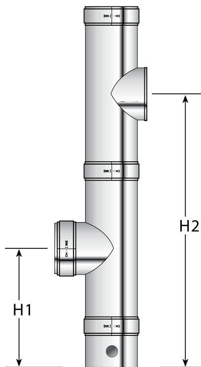
Grīdas montāža
